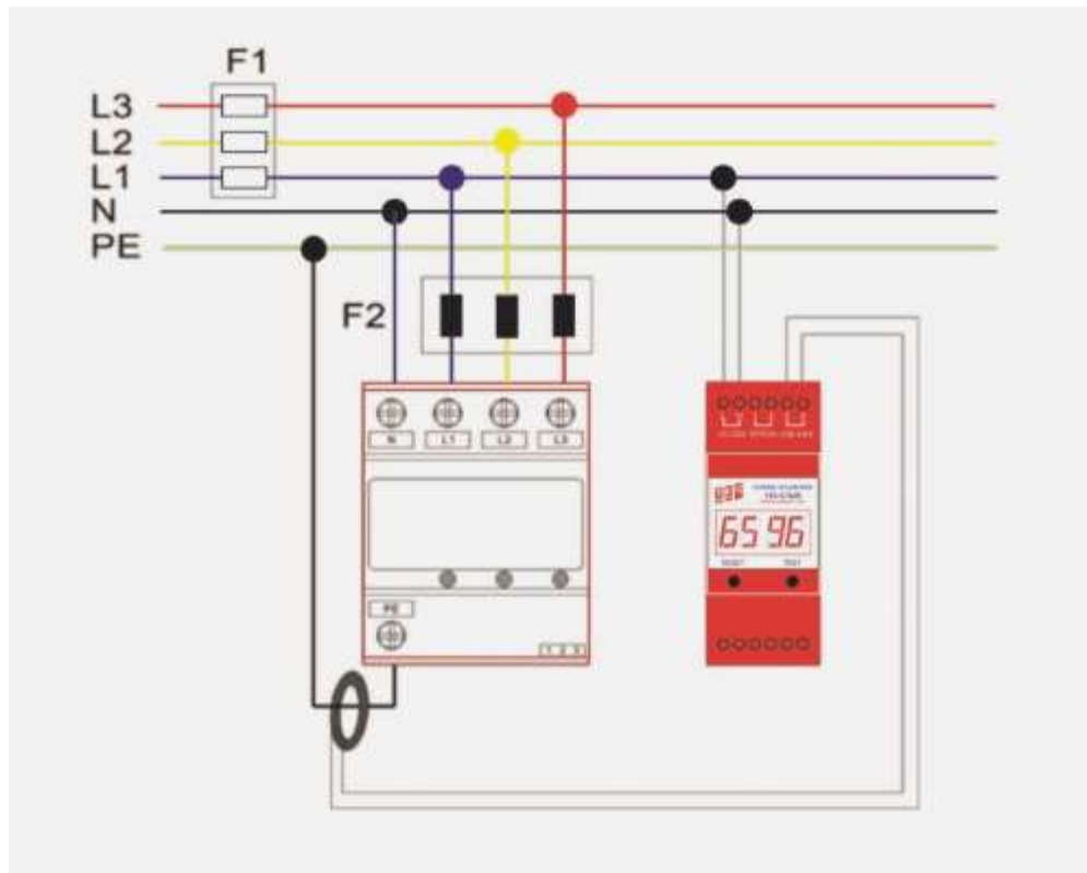
Sơ đồ đấu nối Bộ đếm sét TEC CTL06
